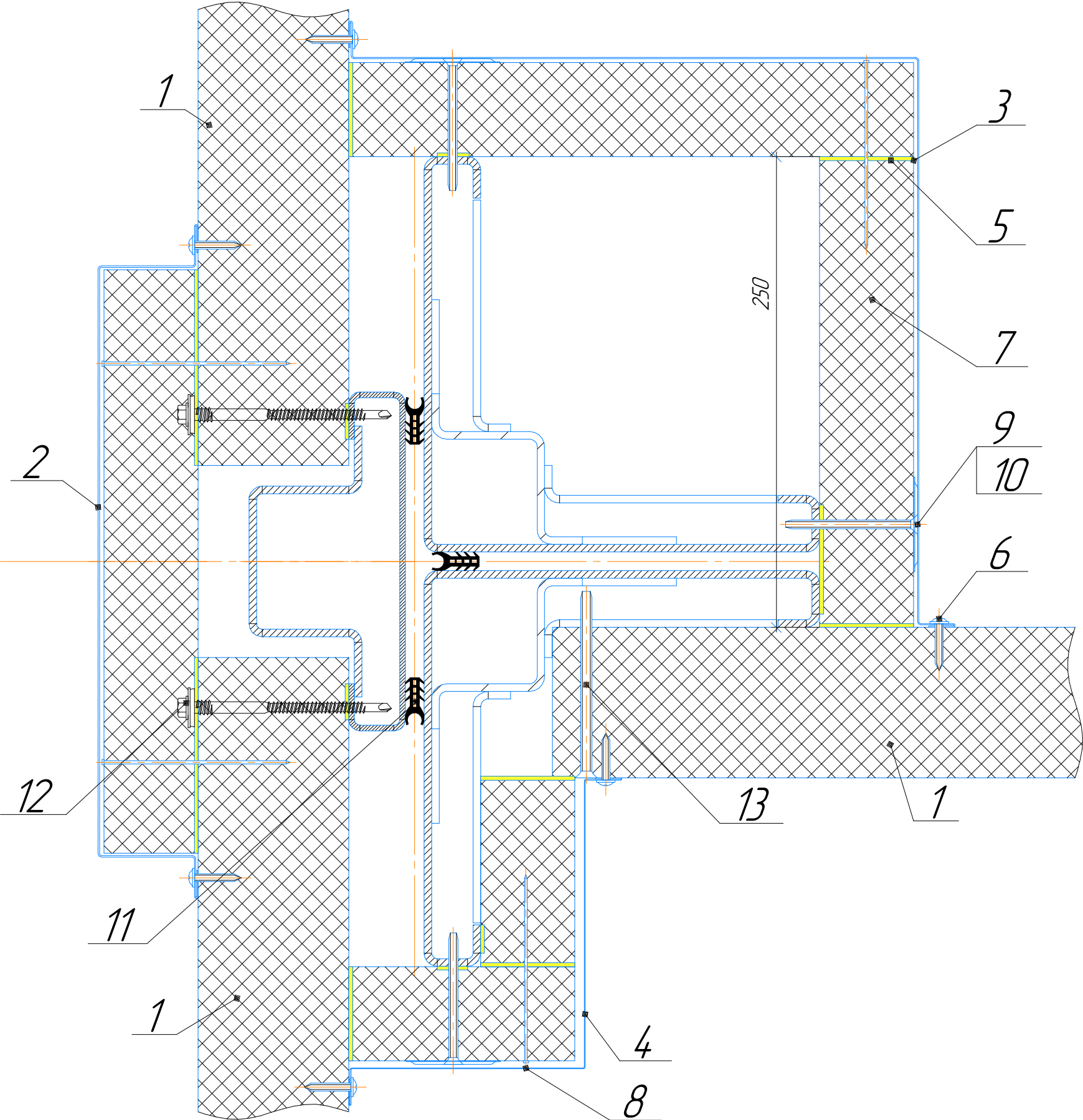
Узел сборки доборных элементов №163
