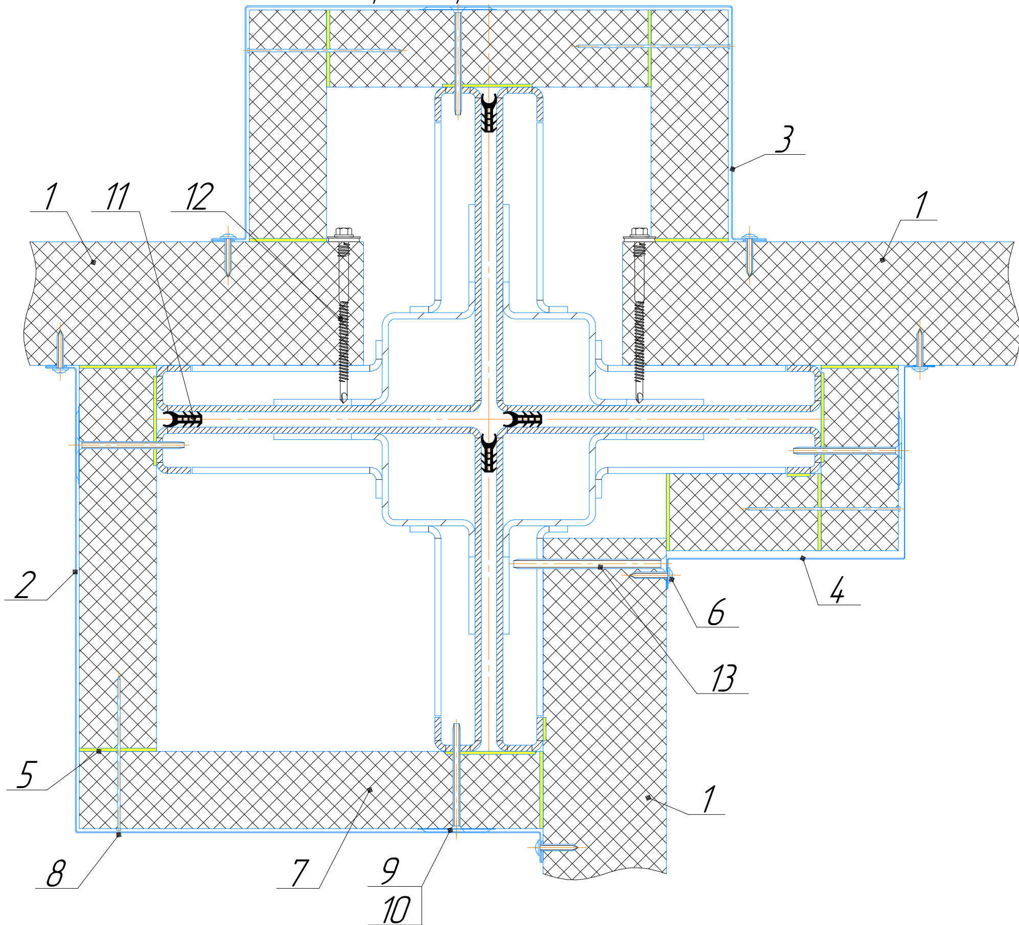
Узел сборки доборных элементов №157
