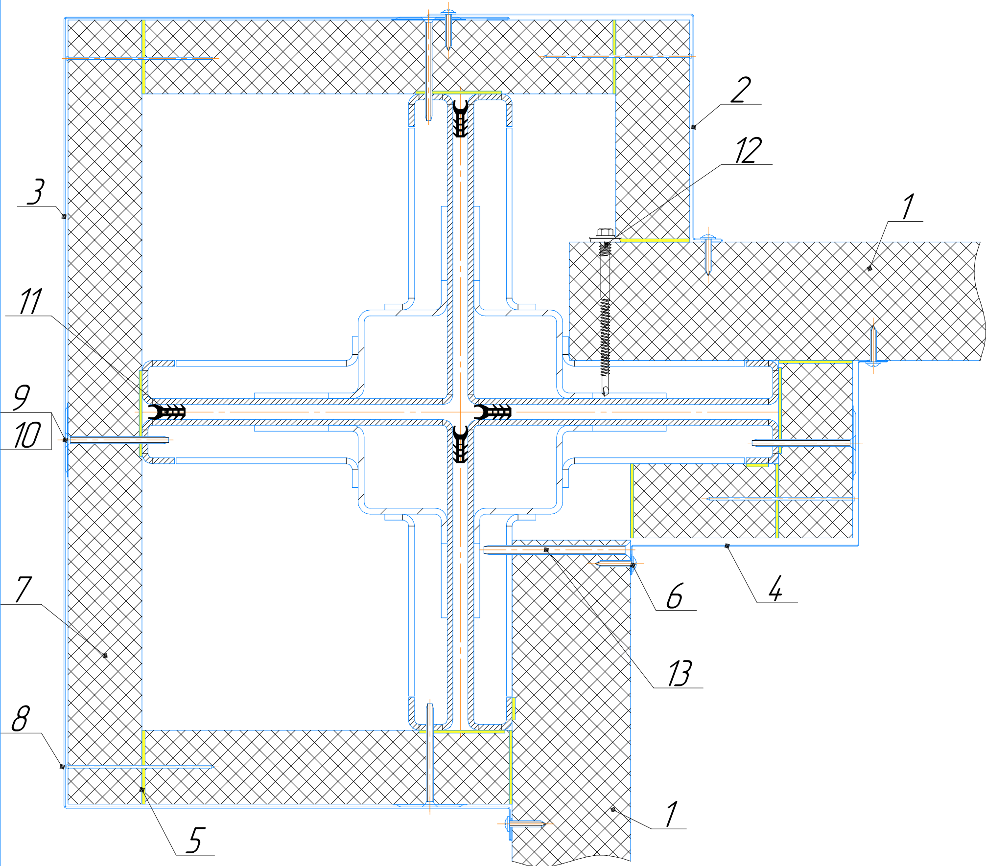
Узел сборки доборных элементов №158
