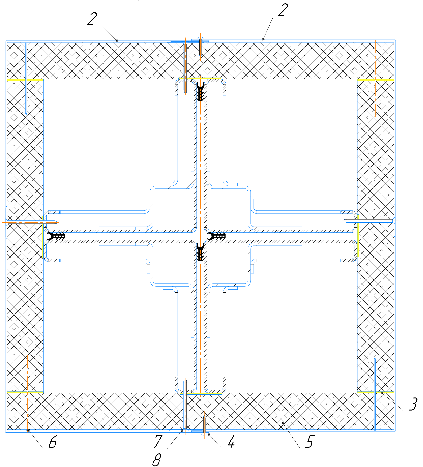
Узел сборки доборных элементов №153
