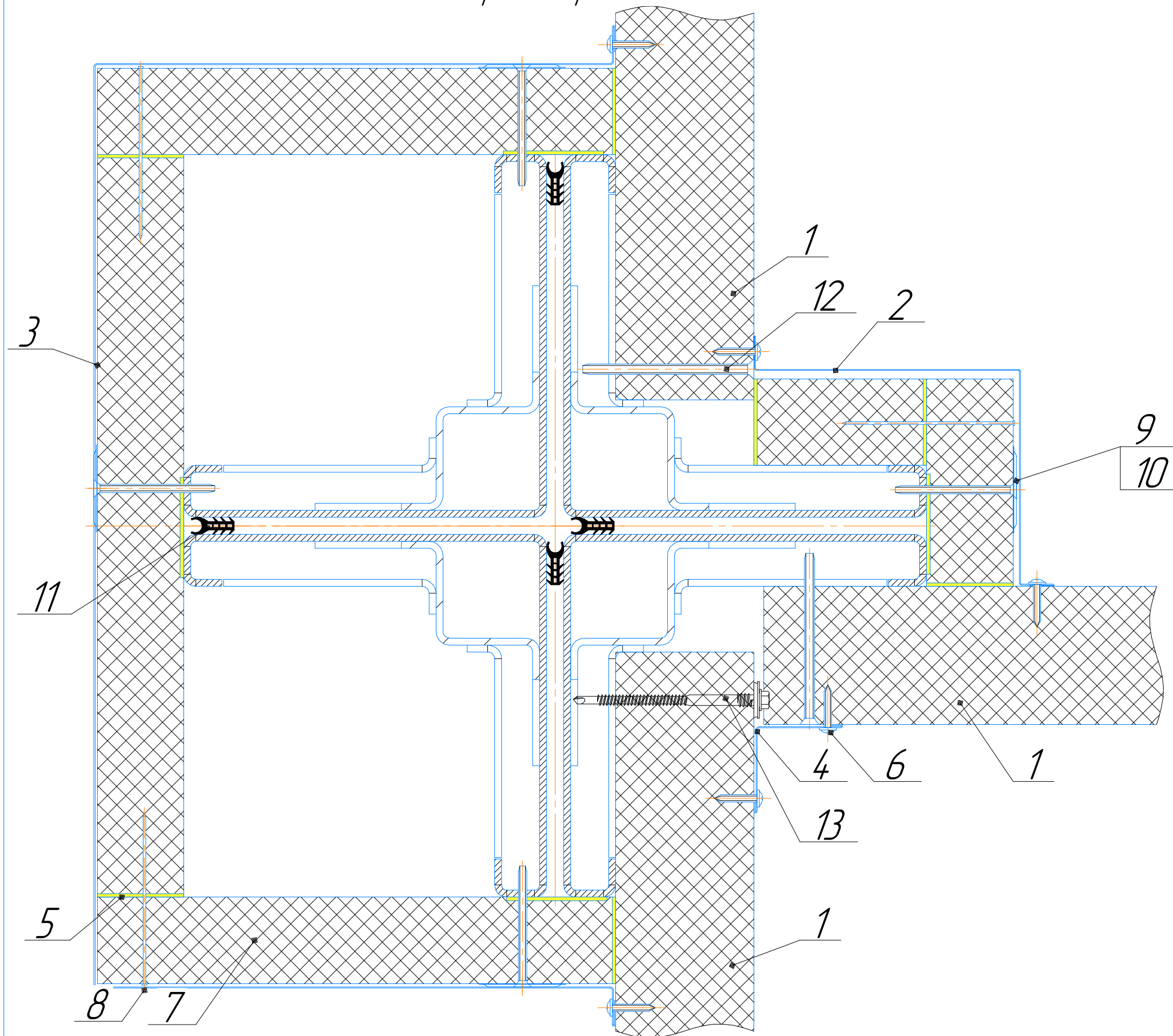
Узел сборки доборных элементов №155
